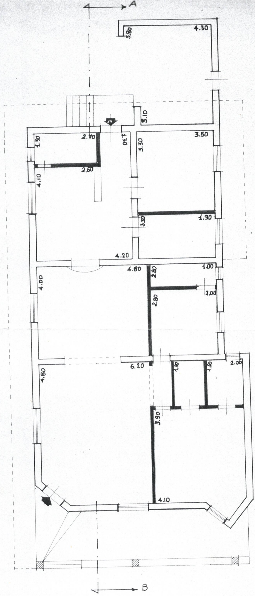
PIANTA PIANO TERRA RAPP. 1:100
